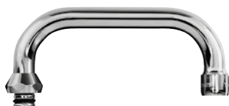
U-Rohrauslauf schwenkbar, Anschlussverschraubung IG3/4", mit Luftsprudler M22x1, Ausladung 200 mm
